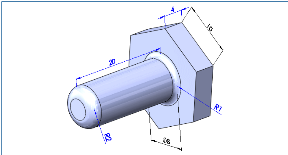
Perno
